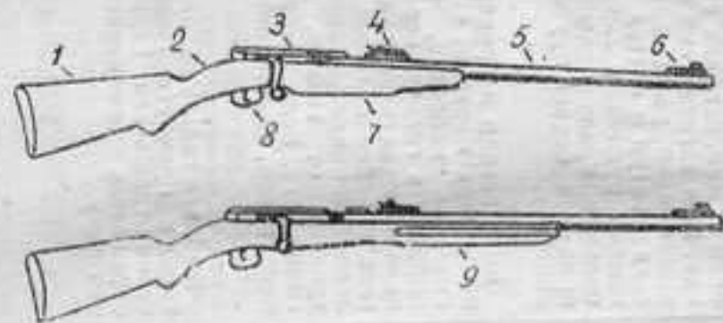
Рис. 4. Малокалиберные винтовки ТОЗ-8 и ТОЗ-9: 1—приклад; 2—шейка приклада; 3—ствольная коробка; 4—прицел; 5—ствол; 6—мушка; 7 и 9—ложа; 8—спусковая скоба.
